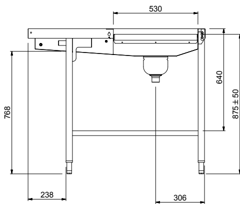
Zij aanzicht
