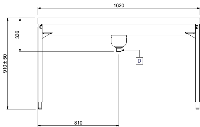
Zij aanzicht
